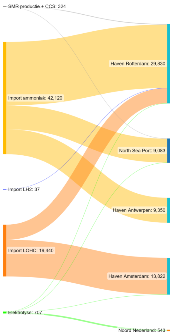
Figuur B4. Import van waterstofdragers en productie van waterstof in variant 3 (in kt H 2,eq ).
