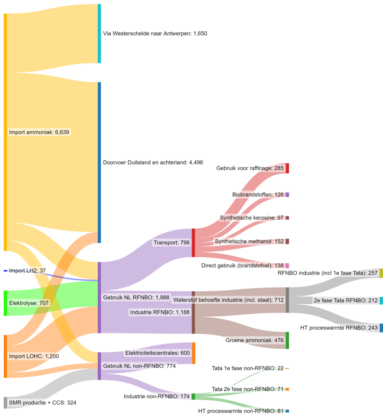
Figuur 7. Vraag en aanbod van RFNBO en koolstofarme waterstof voor variant 3 (in kt H 2,eq ).
