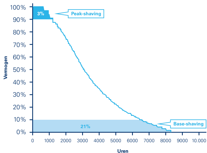
Figuur 19 Vermogensduurkromme van een offshore windturbine, inclusief peak-shaving en base-shaving.
