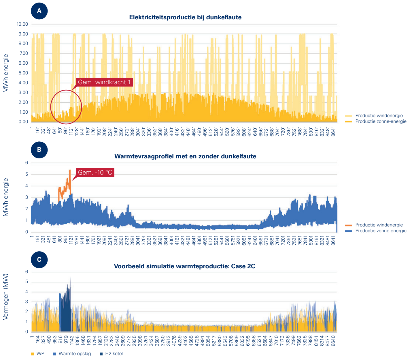
Figuur 8 Bovenstaande grafieken geven respectievelijk de elektriciteitsproductie van zon- en windenergie (a), de warmtevraag (b) en de warmteproductie (c) weer voor de gesimuleerde Dunkelflaute.
