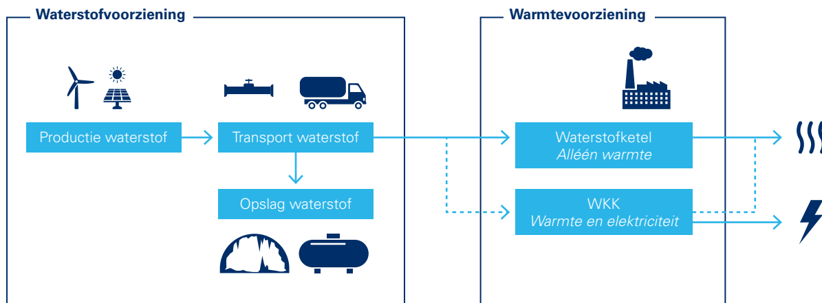
Figuur 18 De voorzieningsketen voor waterstof en de warmtevoorziening op waterstof
