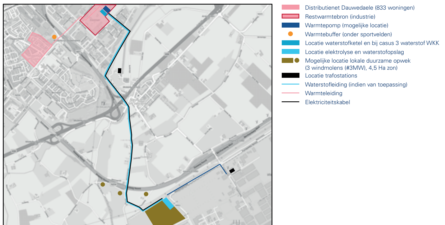
Figuur 5 Schematische weergave van mogelijke technische configuratie van een duurzaam warmtenet in Dauwendaele. indicatieve locaties voor wind- en zonne-energie.
